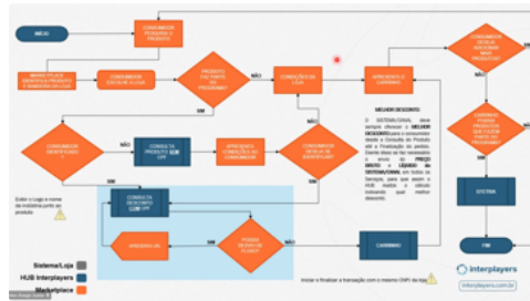
Fluxo de vitrine e compra
