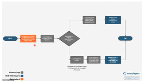
Fluxo de pagamento
